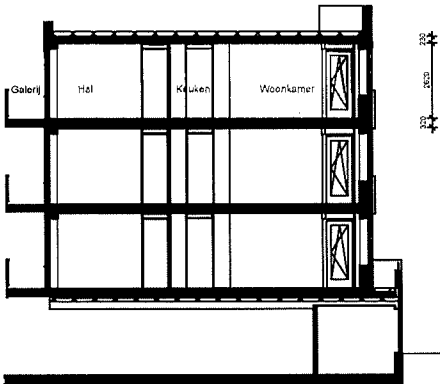
Doorsnede
