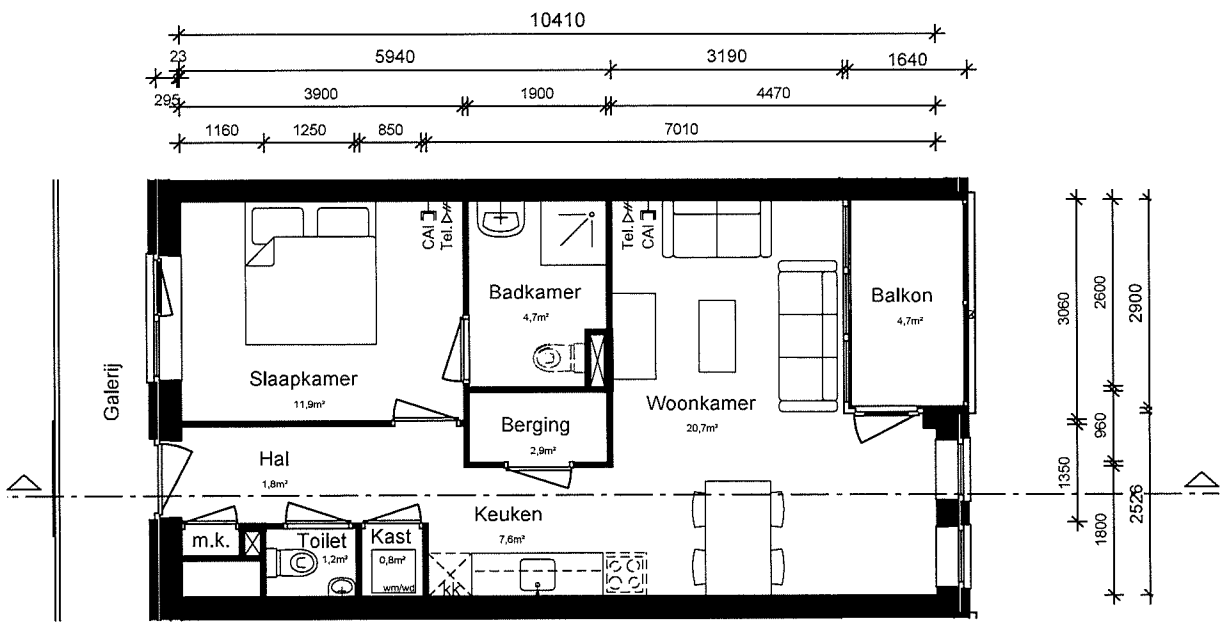
Plattegrond
