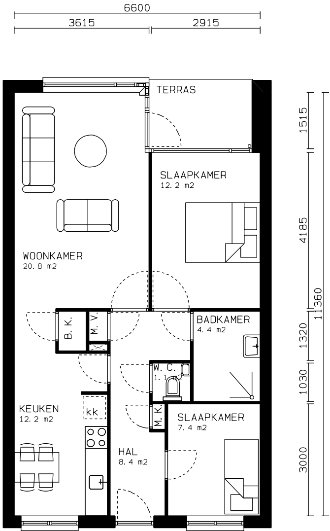
BEGANE GROND
