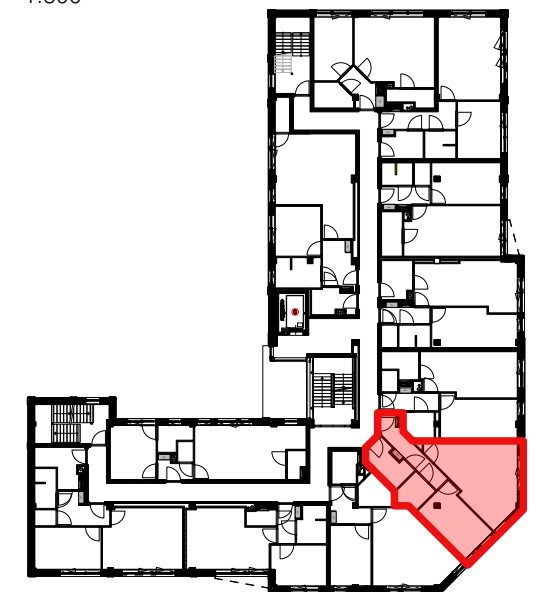
Overzicht plattegrond - 3e verdieping 1:500
