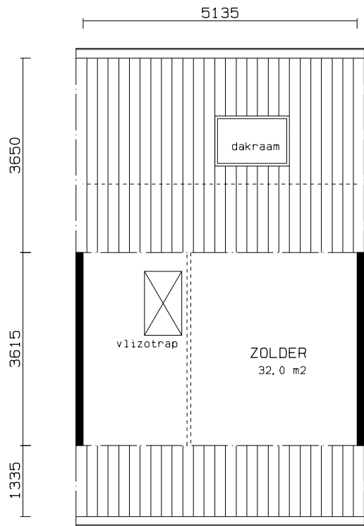
2e VERDIEPING
