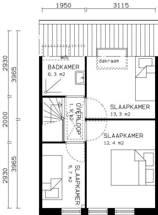
1e VERDIEPING
