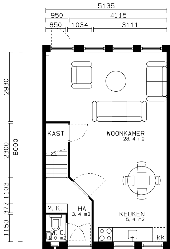
BEGANE GROND
