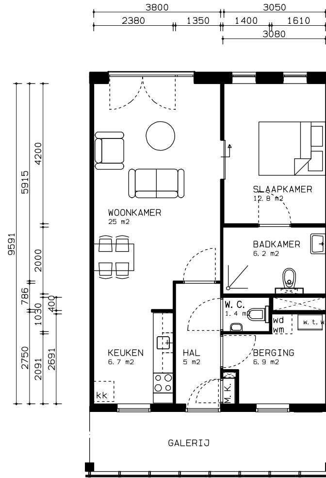
2e VERDIEPING
