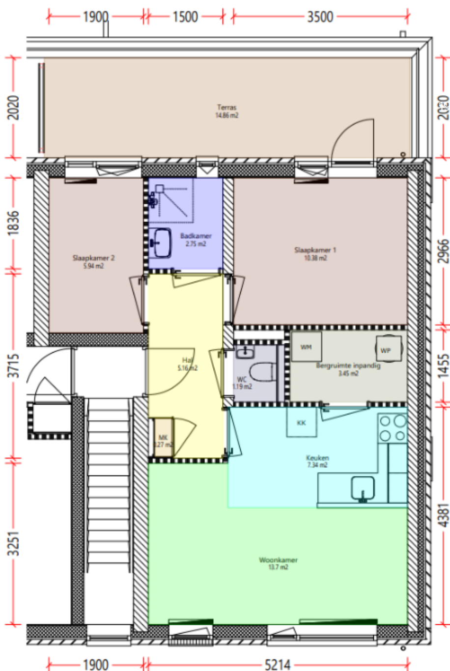
Eerste verdieping
