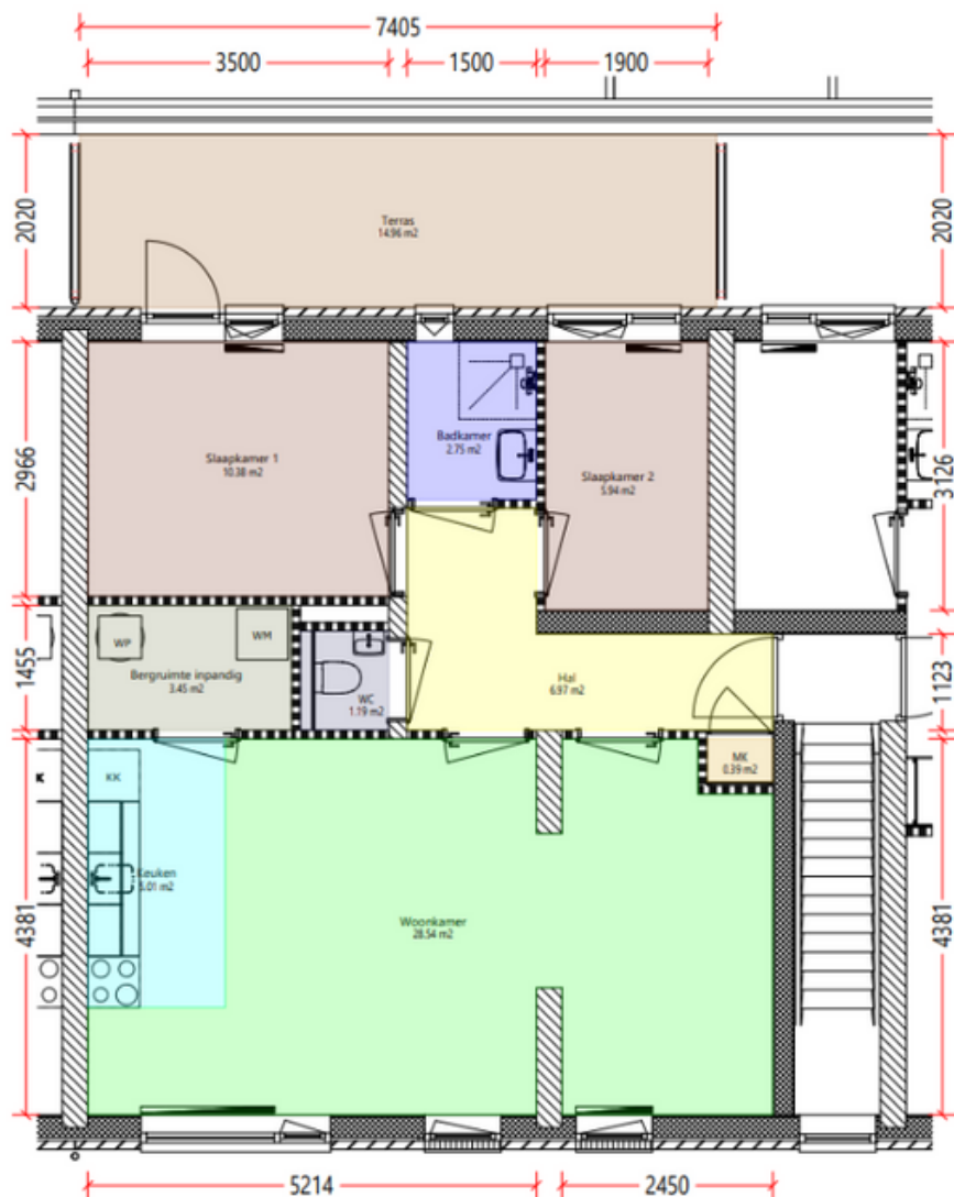
Eerste verdieping
