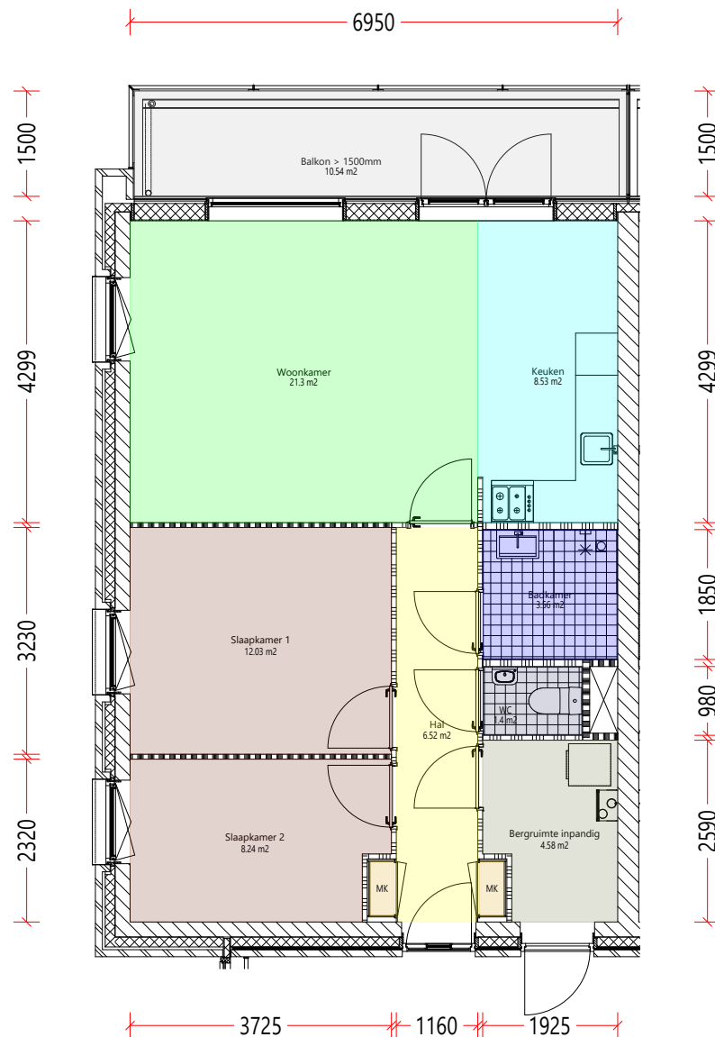
Verdieping_3e
